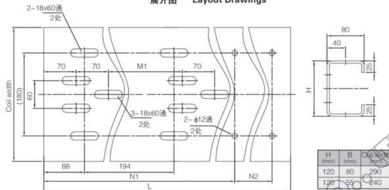
展开图 Layout Drawings
